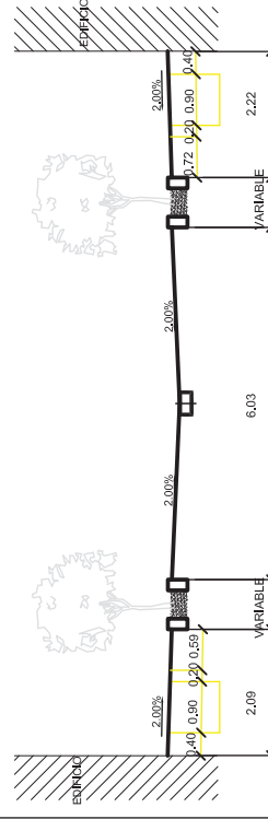
SECCIÓN A-A
